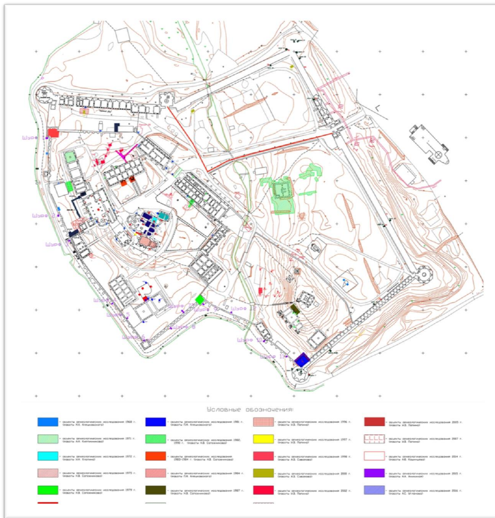
Рисунок 1. Общий план археологии Кирилло-Белозерского монастыря. Автор – Угланов А.С.
